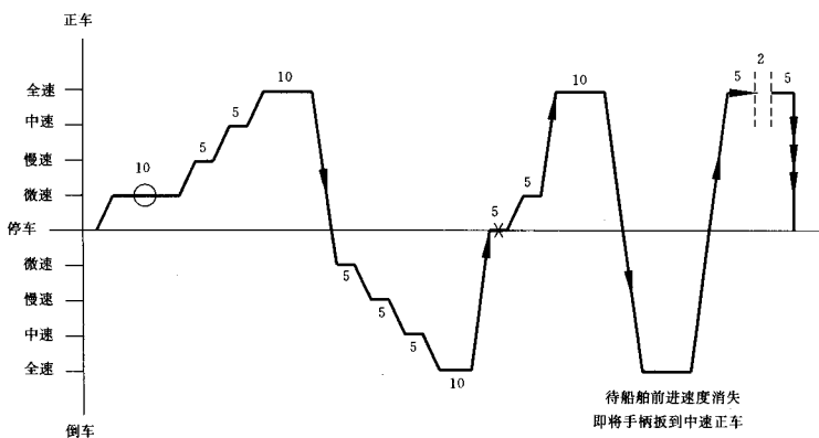
图2 柴油机动力可调螺距螺旋桨推进装置单手柄控制系统试验程序
